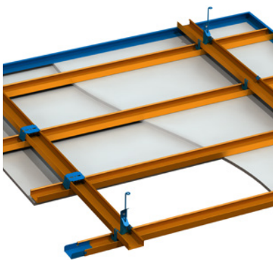
Runkojärjestelmät
